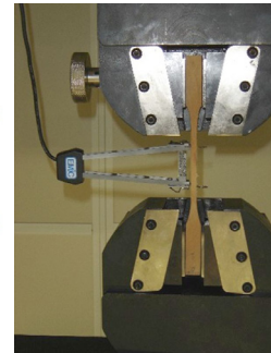
Fig. 4: Tensile test.
